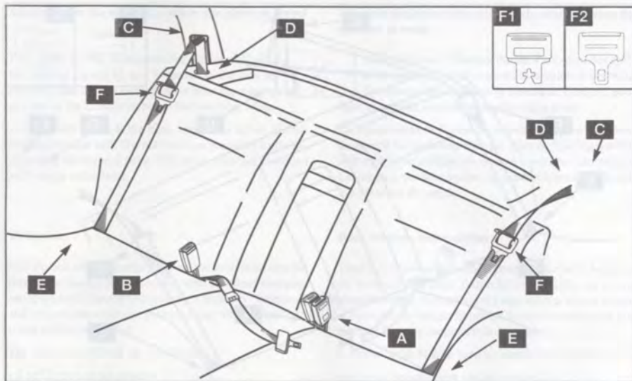
ENG: Rear seat, 200 series sedan. FRA: Banquette arrière, berline des séries 200.
