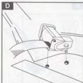
ENG: Retractor, rear shelf. FRA: Enrouleur de ceinture de sécurité, plage arrière.
